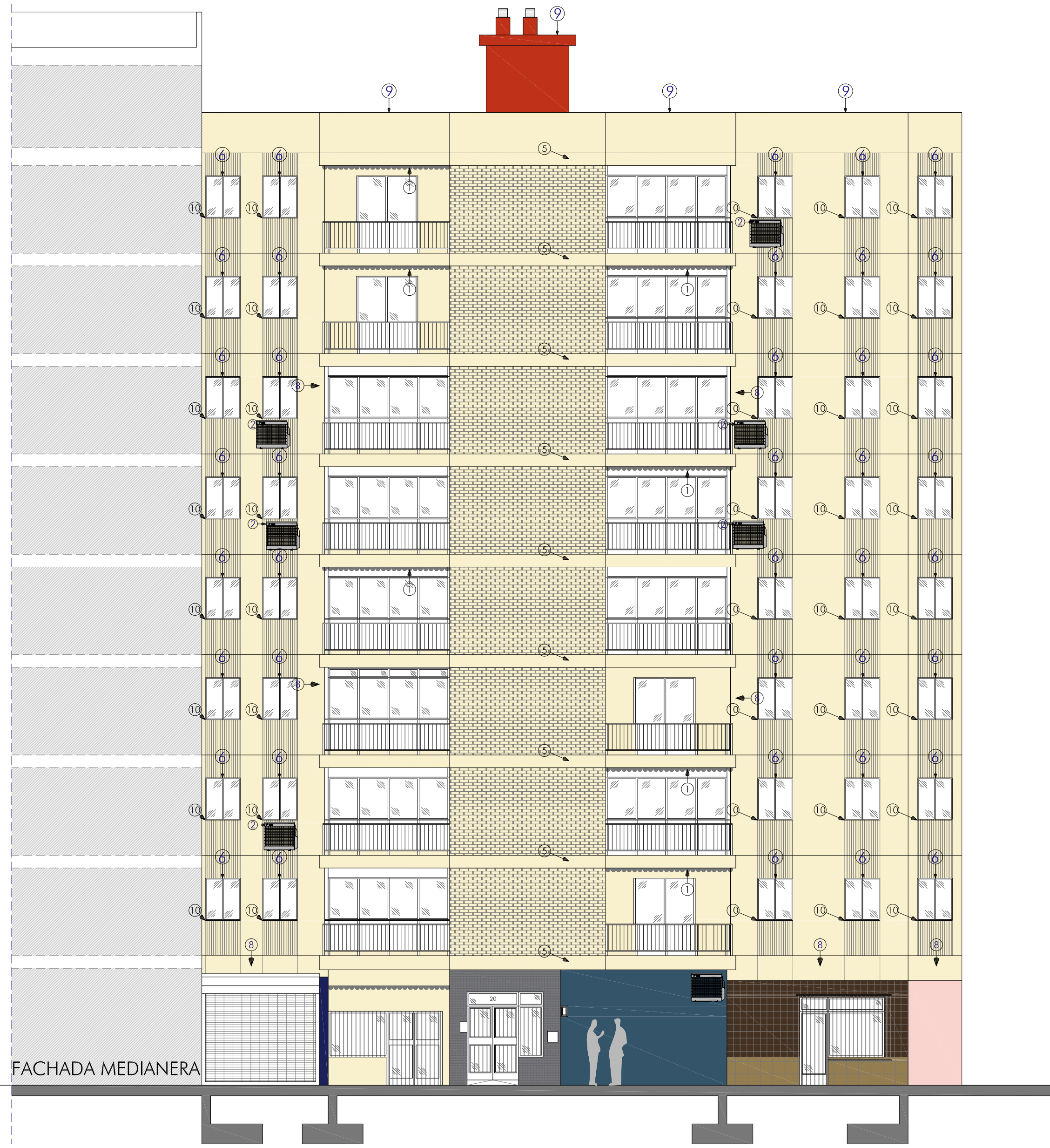
ALZADO 1 (NOROESTE)
