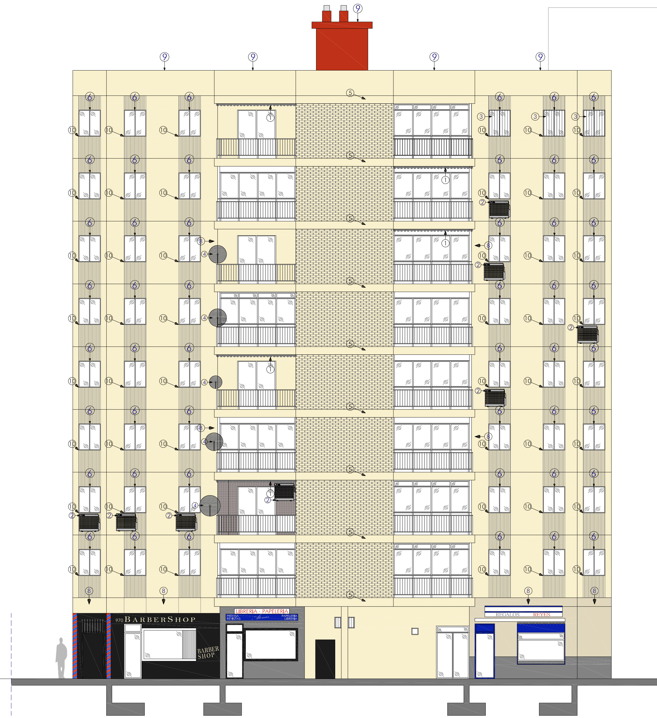
ALZADO 2 (SURESTE)
